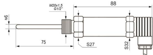
Рисунок 1 – Термопреобразователь с цифровым выходом T.Pt – RS – DIN – 6 – 75 – (-70/+200)
